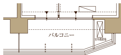
D1' type 部分図
