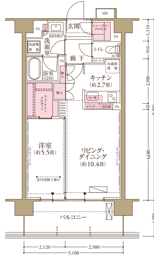
C1' typeはC1 type(5号室系統)の反転になります。 上記図面はC1 typeになります。
